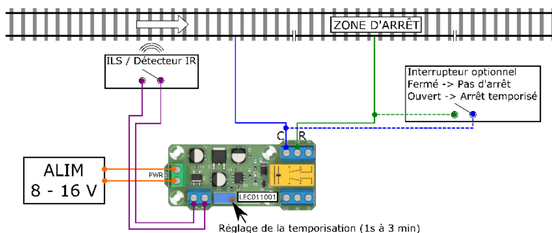
Figure 8 – Arrêt temporisé automatique en gare (version Analogique)
