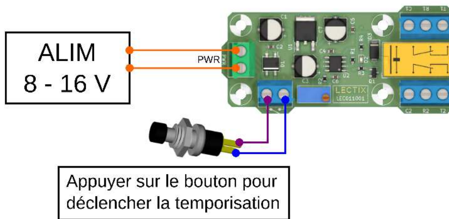
Figure 1 – Schéma de câblage du module.
