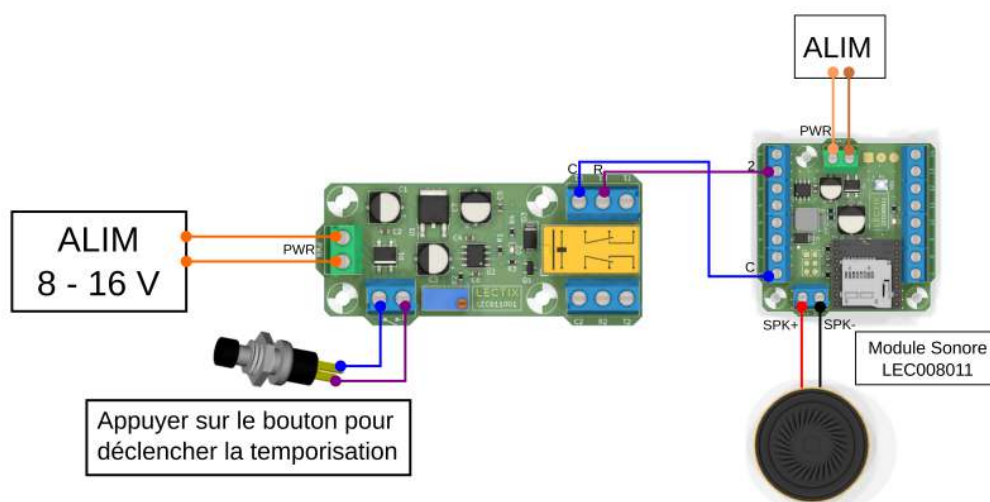
Figure 6 – Activation d'un son à la fin du délais réglé.
