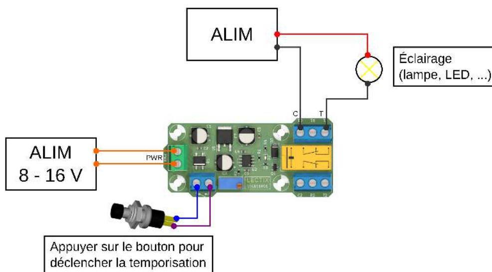
Figure 5 – Activation d'un éclairage pour une durée déterminée.
