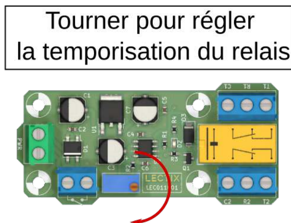
Figure 3 – Réglage de la temporisation.
