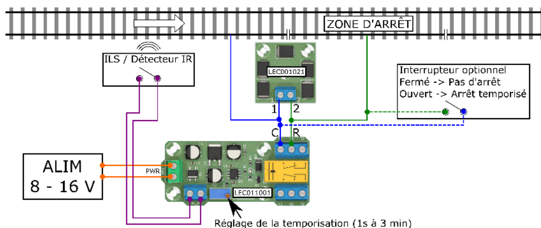
Figure 7 – Arrêt temporisé automatique en gare (version DCC)
