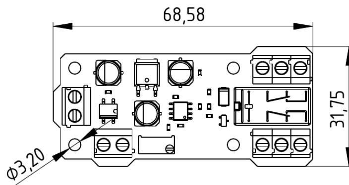
Figure 4 – Dimensions du module (toutes les côtes sont données en mm).
