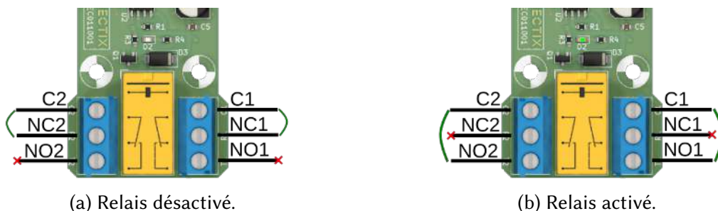
Figure 2 – Description des contacts inverseurs du relais.
