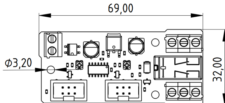
Figure 1 – Dimensions du module (toutes les côtes sont données en mm).
