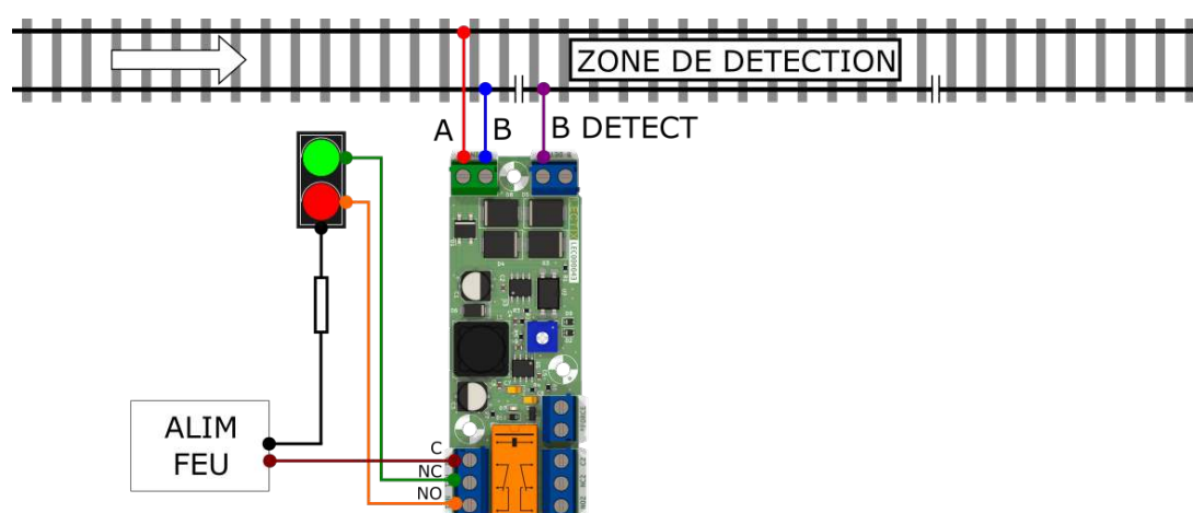
Figure 5: Branchement d'un feu bicolore.
