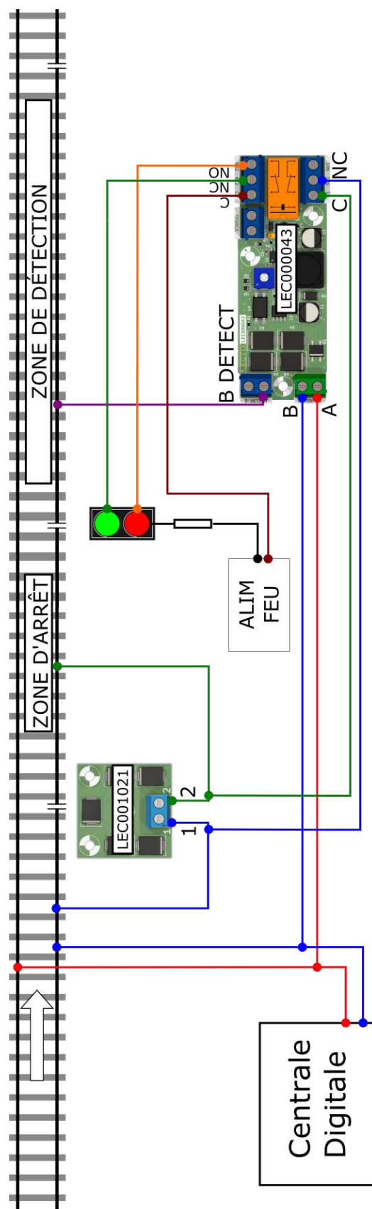
Figure 9: Ajout d'un feu bicolore dans un montage de type cantonnement.
