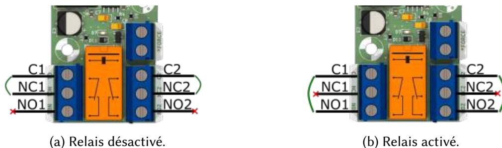
Figure 2: Description des contacts inverseurs du relais.
