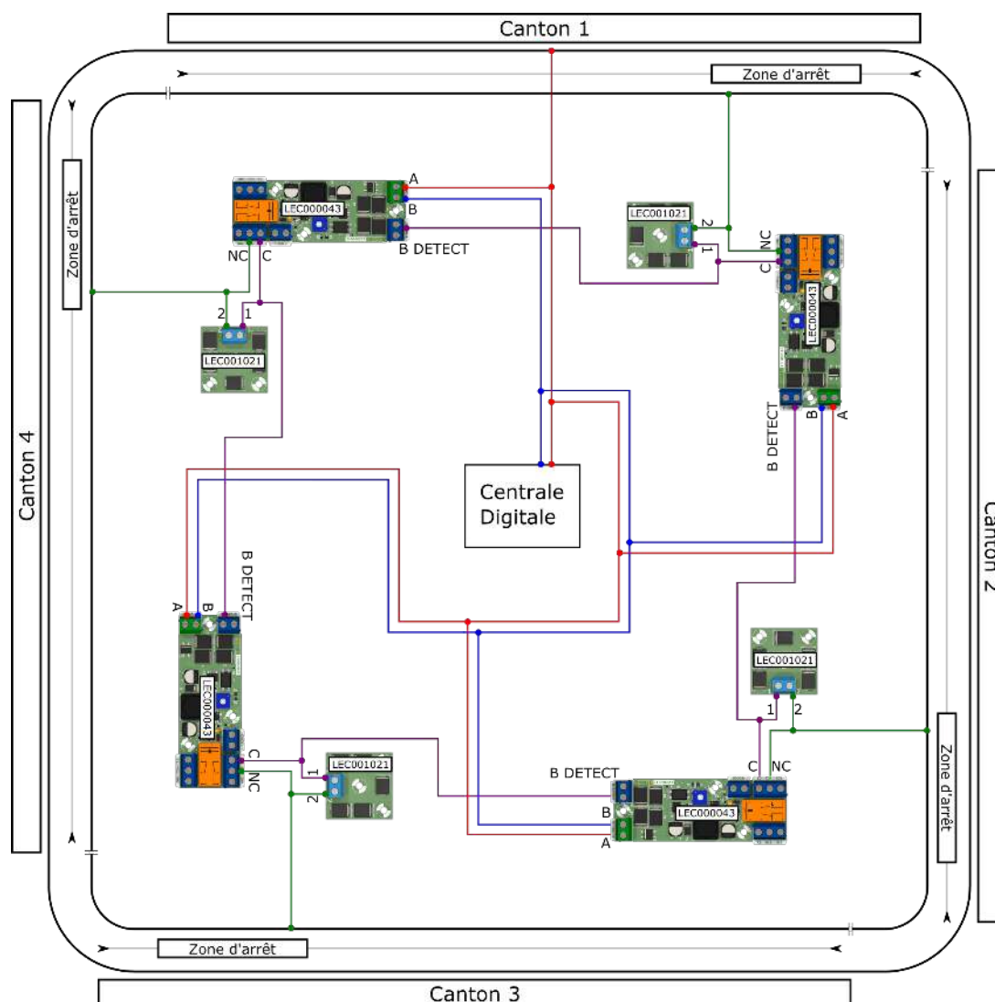
Figure 13: Cantons successifs sans zones de roulage.
