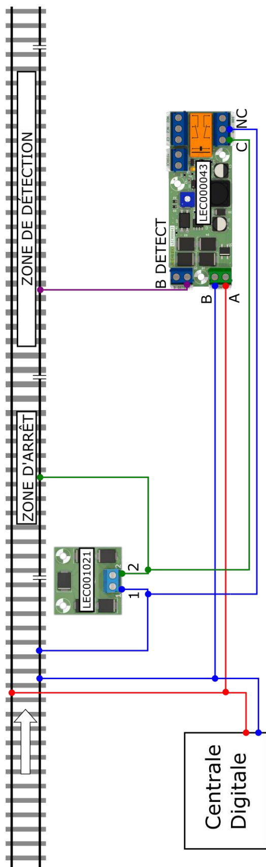
Figure 7: Protection d'un tronçon avec arrêt automatique.
