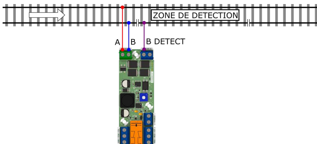
Figure 1: Schéma de câblage du module.
