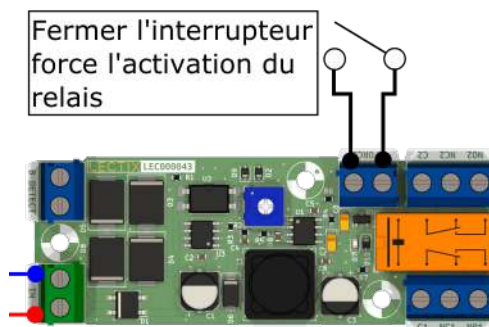
Figure 3: Forçage de l'activation du relais.
