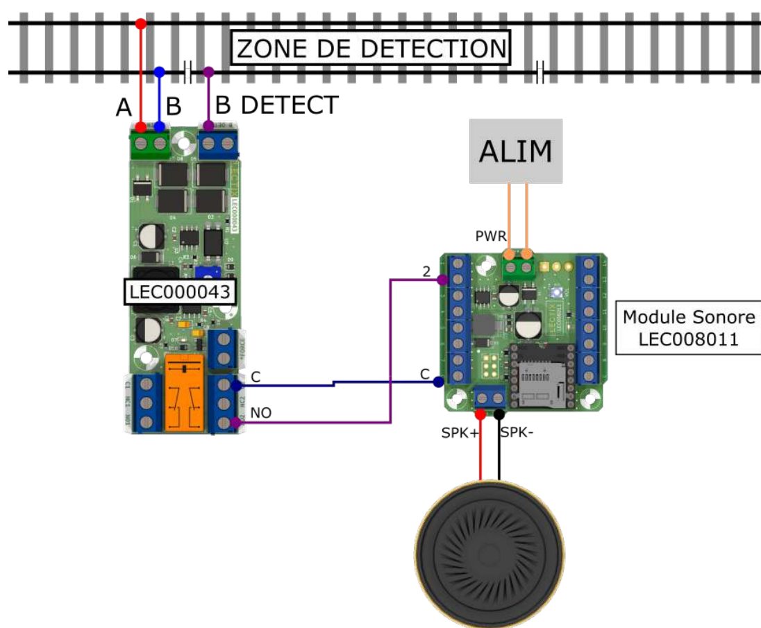
Figure 6: Déclenchement d'un signal sonore.
