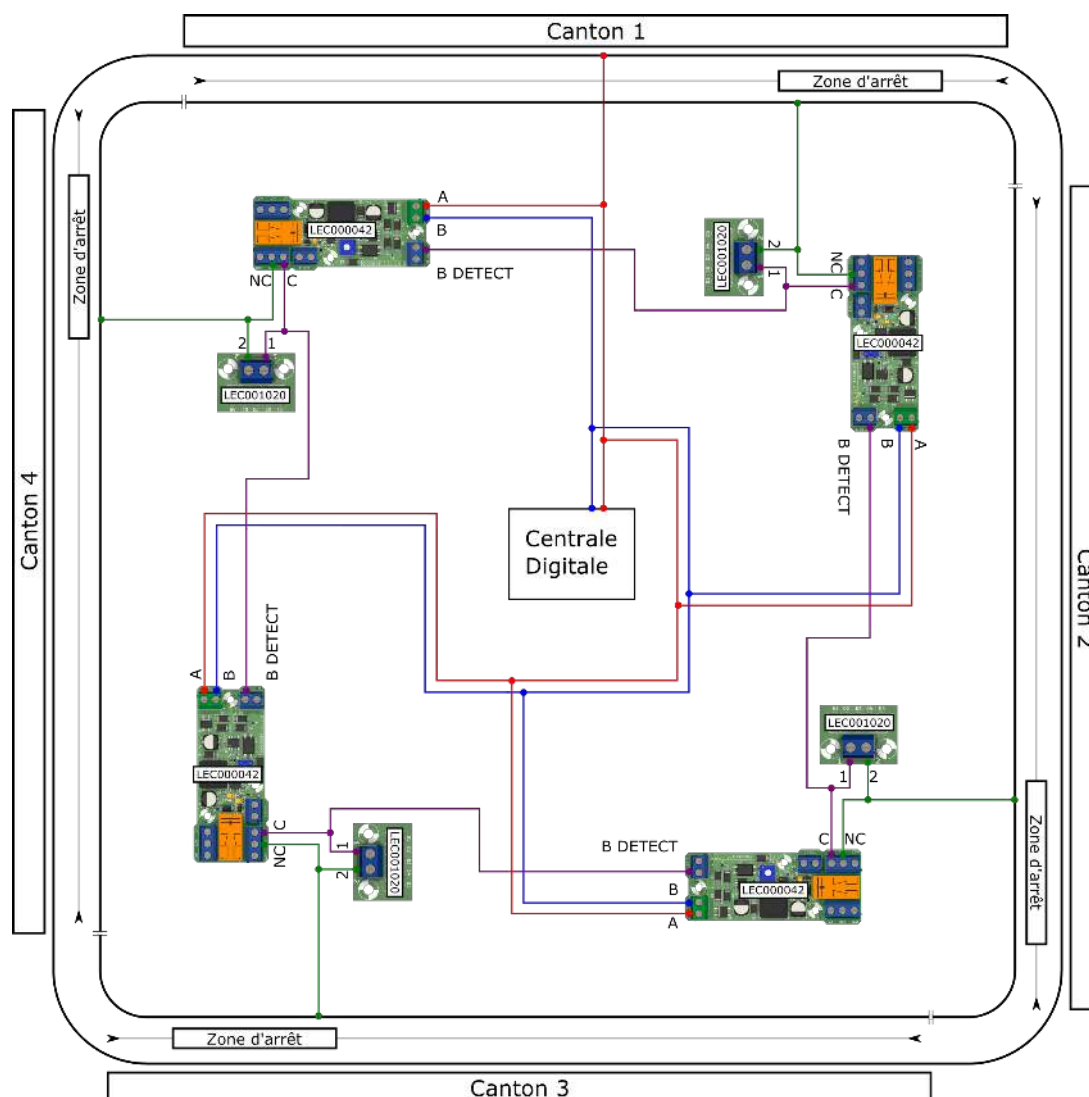
Figure 14: Cantons successifs sans zones de roulage.
