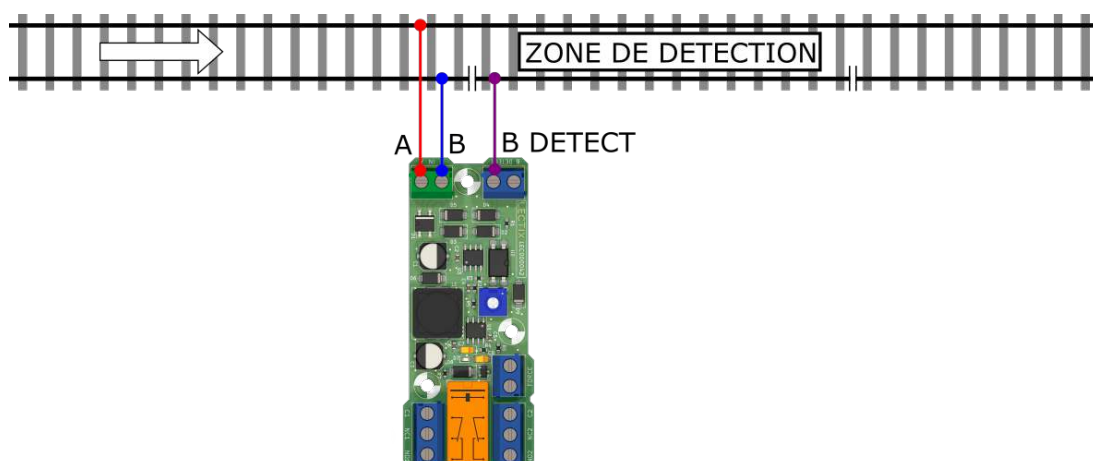
Figure 2: Schéma de câblage du module.
